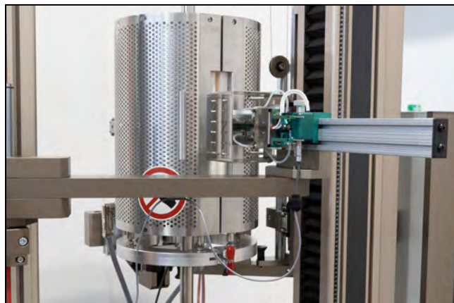
Kontaktierendes Hochtemperatur-Extensometer bis 1.600°C
